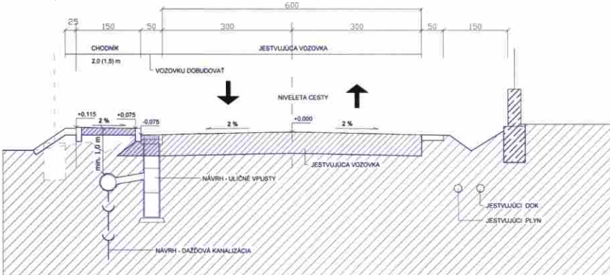
Priečny rez navrhovanou vozovkou v obci
