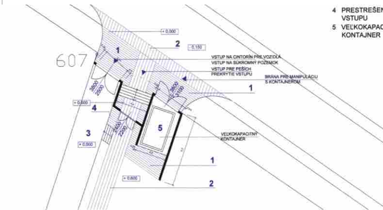
Návrh úpravy centrálneho vstupu na cintorín
